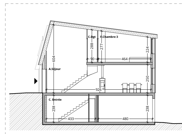
COUPE TRANSVERSALE 1:200
