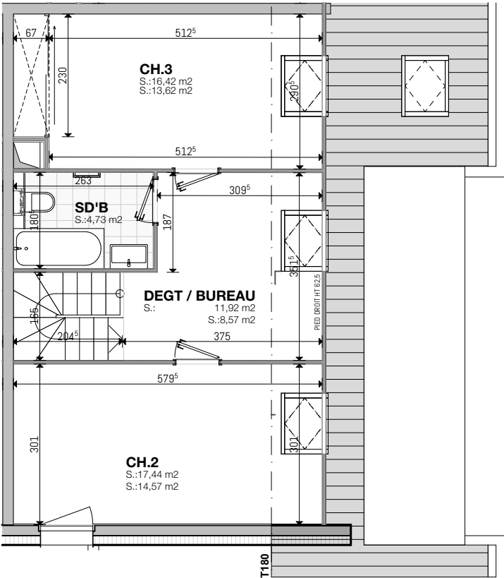
3ème ÉTAGE
