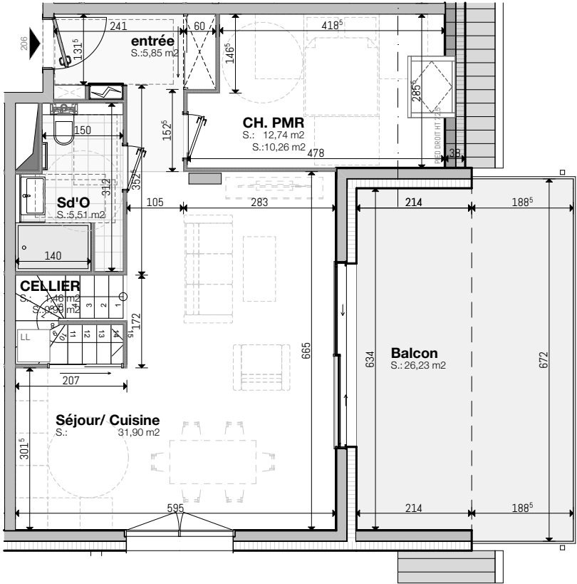
2ème ÉTAGE
