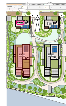
Plan de masse
